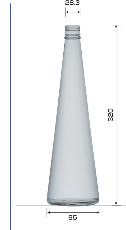
AK-NS720
