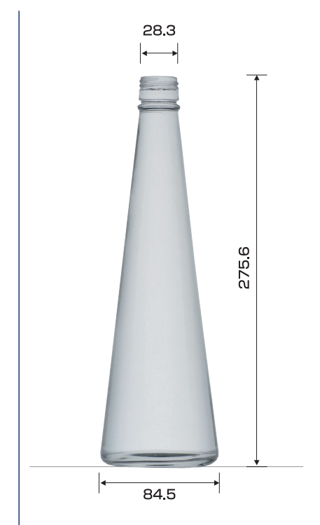
AK-NS500
