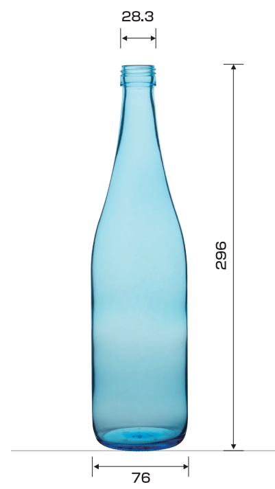
PP30 SW720A
