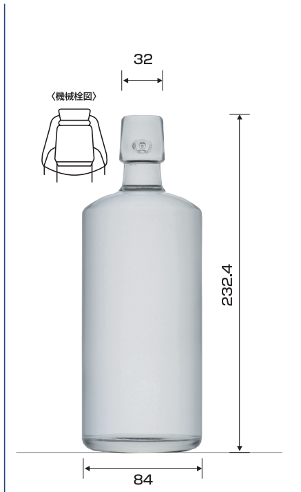
ASP720 (機械栓)
