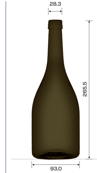
ASC泡盛720
