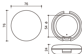
AJ-54 φ (2段) W76.0×D76.0×H24.0
