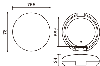
AJ-58 φ (2段) W76.5×D78.0×H24.0
